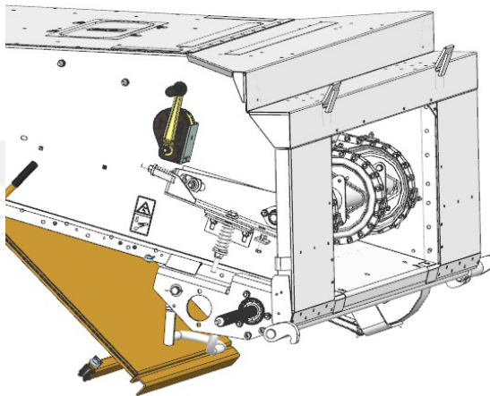
Reinigungsöffnung im Schrägförderschacht
