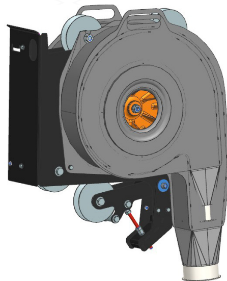
Hochleistungsgebläse für pneumatische Kornförderung
