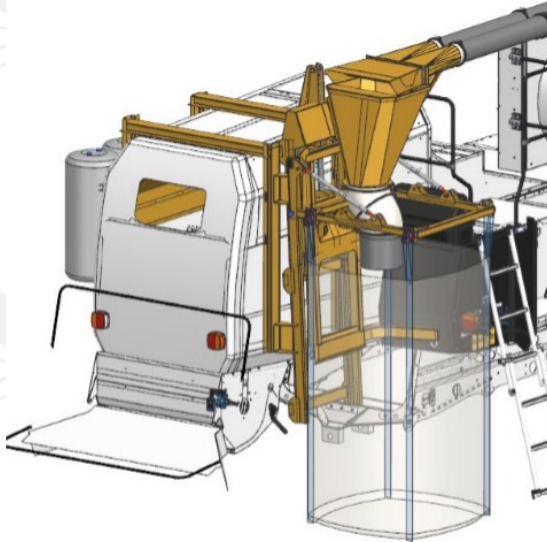
Big-Bag-Abfüllvorrichtung
