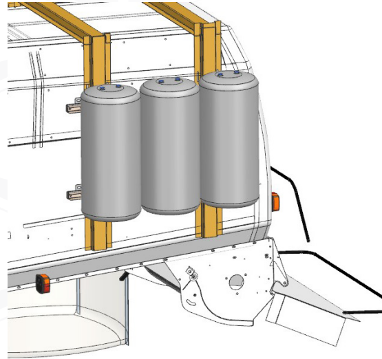
360 l Druckluftbehälter
